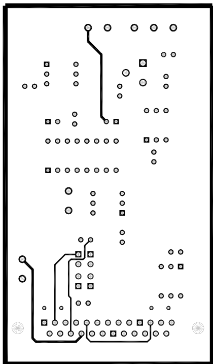
Сторона монтажа
