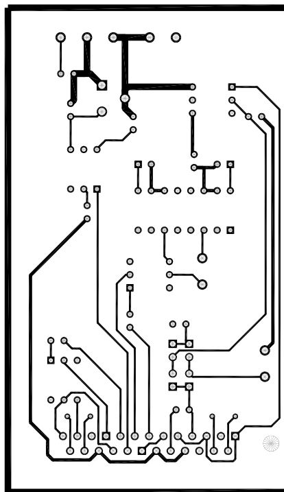
Сторона пайки
