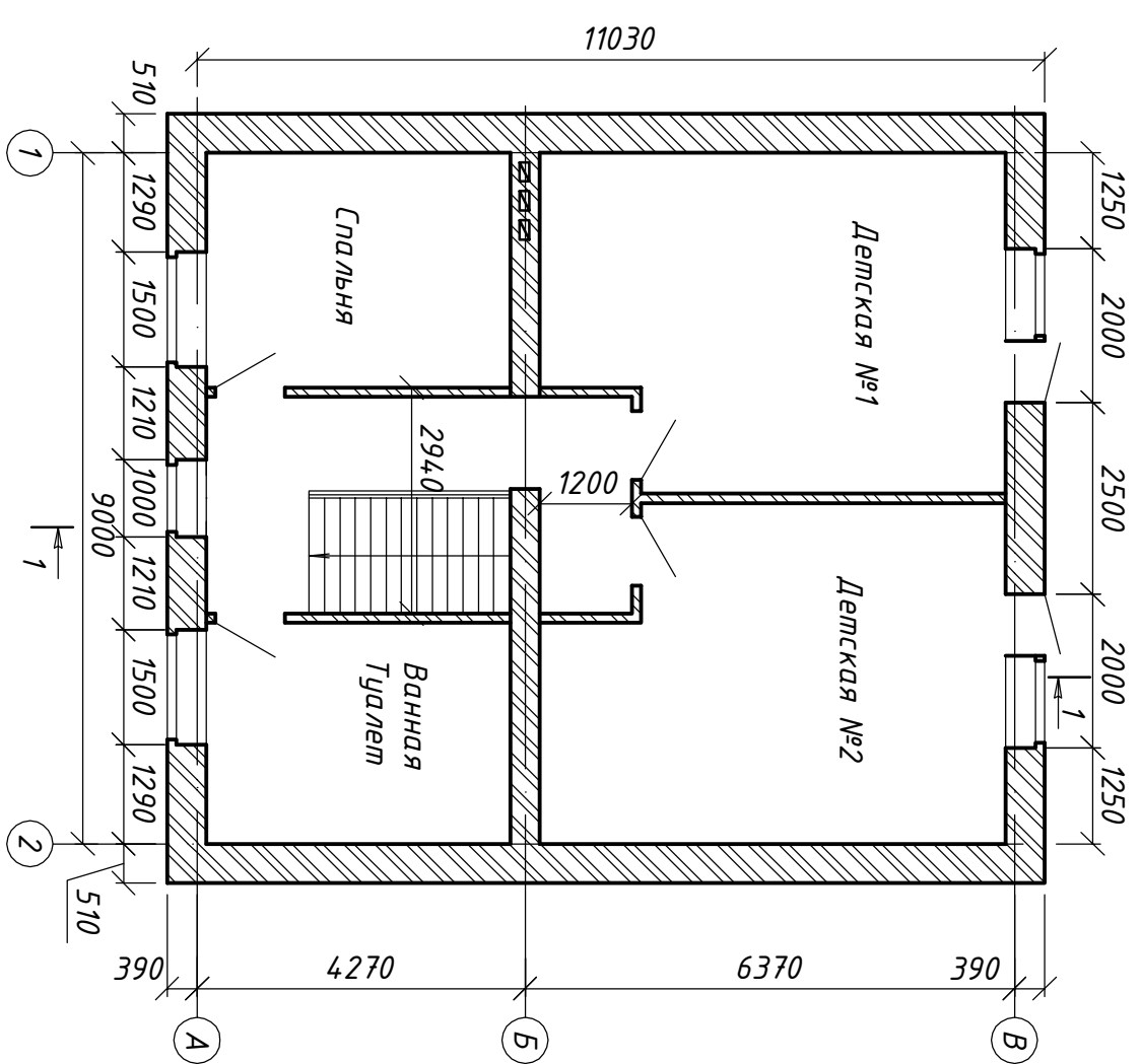
План 2 этажа (1:100)
