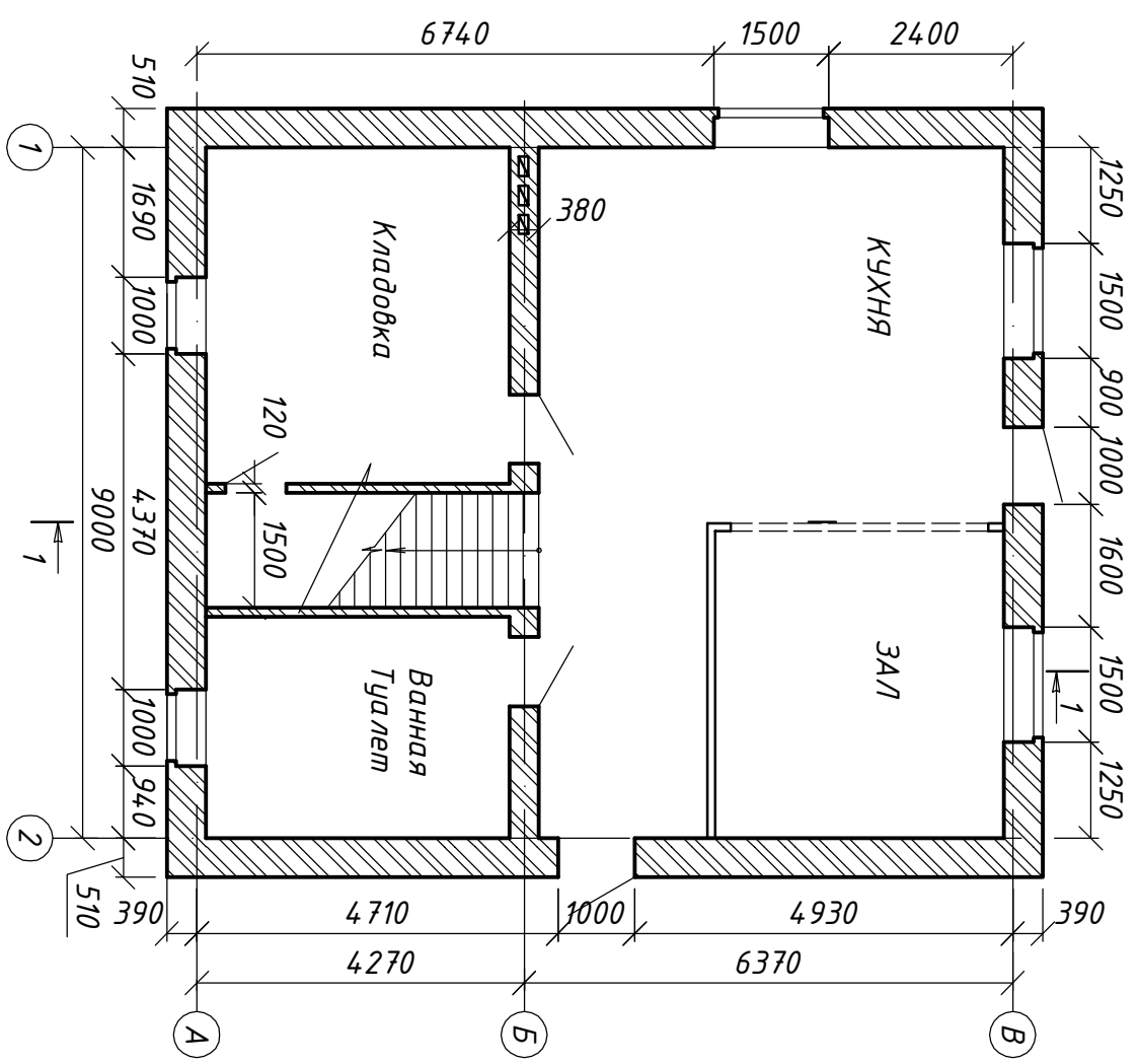
План 1 этажа (1:100)
