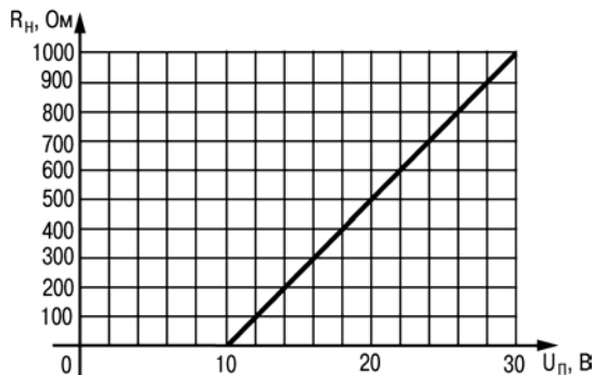
Рис 3.16. График зависимости R_H(U_H)
