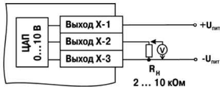
Рис. Б.7. Схема подключения нагрузки к ВУ типа У
