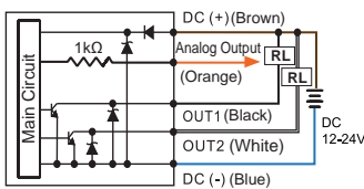
KP43 □ - 010 - □ 2 NPN + Analog Output(1~5V)
