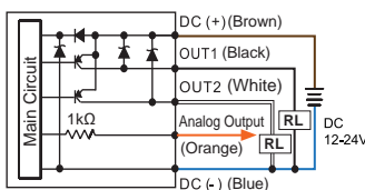
KP43 □ - 030 - □ 2 PNP + Analog Output(1~5V)
